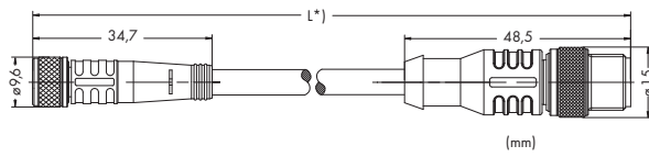
M12 Plug
